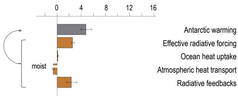
(c) Tropics warming contributions (°C)
